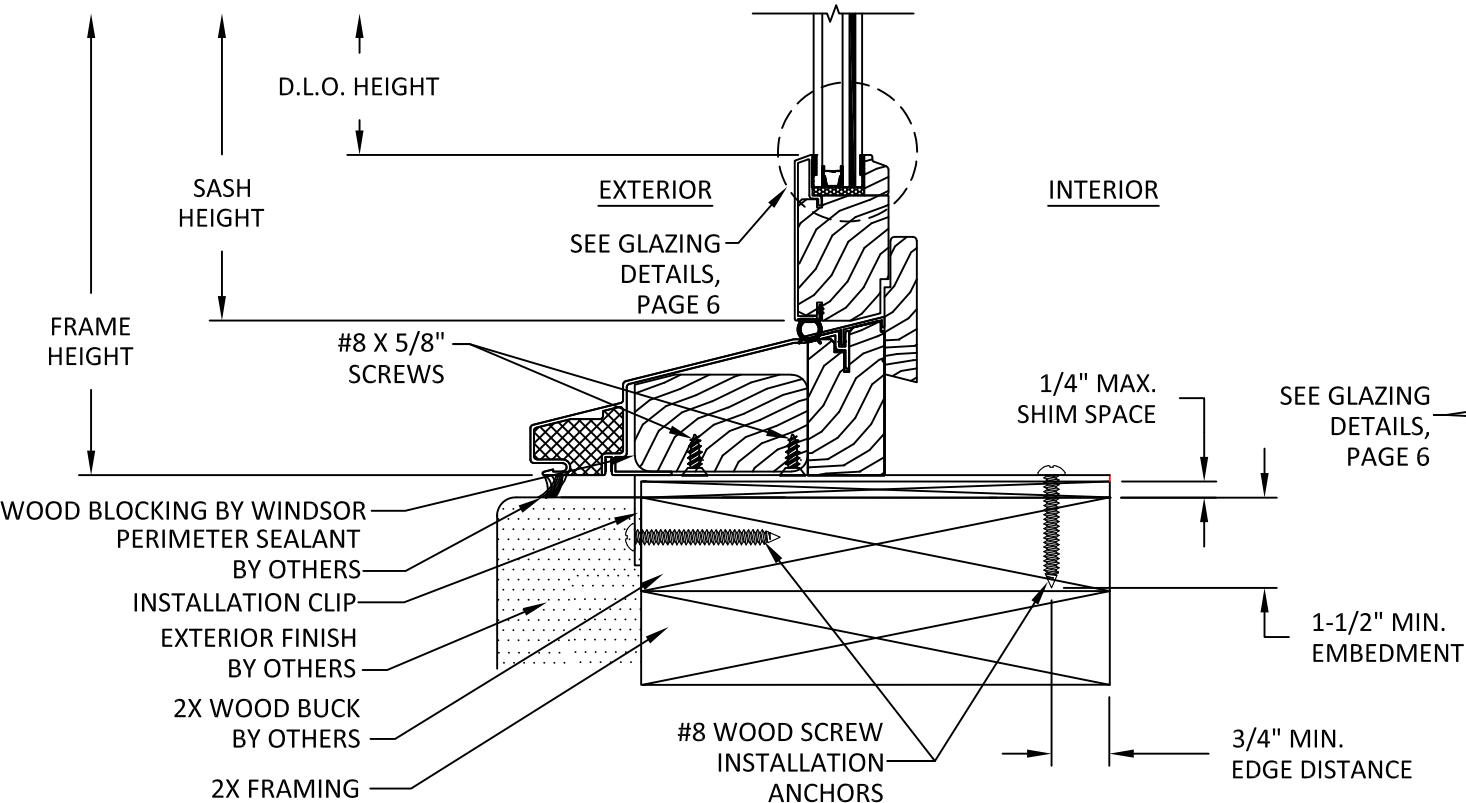
B 3 VERTICAL SECTION DH SILL - 2X WOOD BUCK CLIP INSTALLATION
