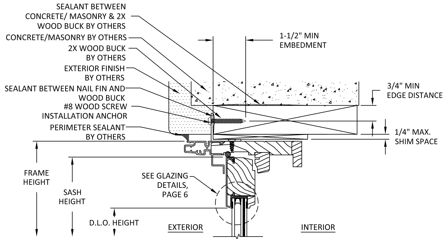
I 5 VERTICAL SECTION DH HEAD - 2X WOOD BUCK NAIL FIN INSTALLATION
