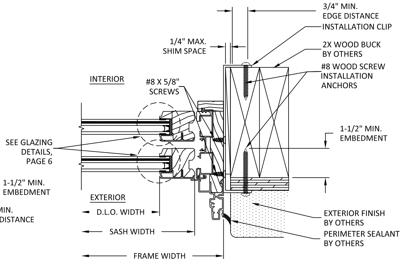
H 4 HORIZONTAL SECTION DH JAMB - 2X WOOD FRAMING STANDARD CLIP INSTALLATION
