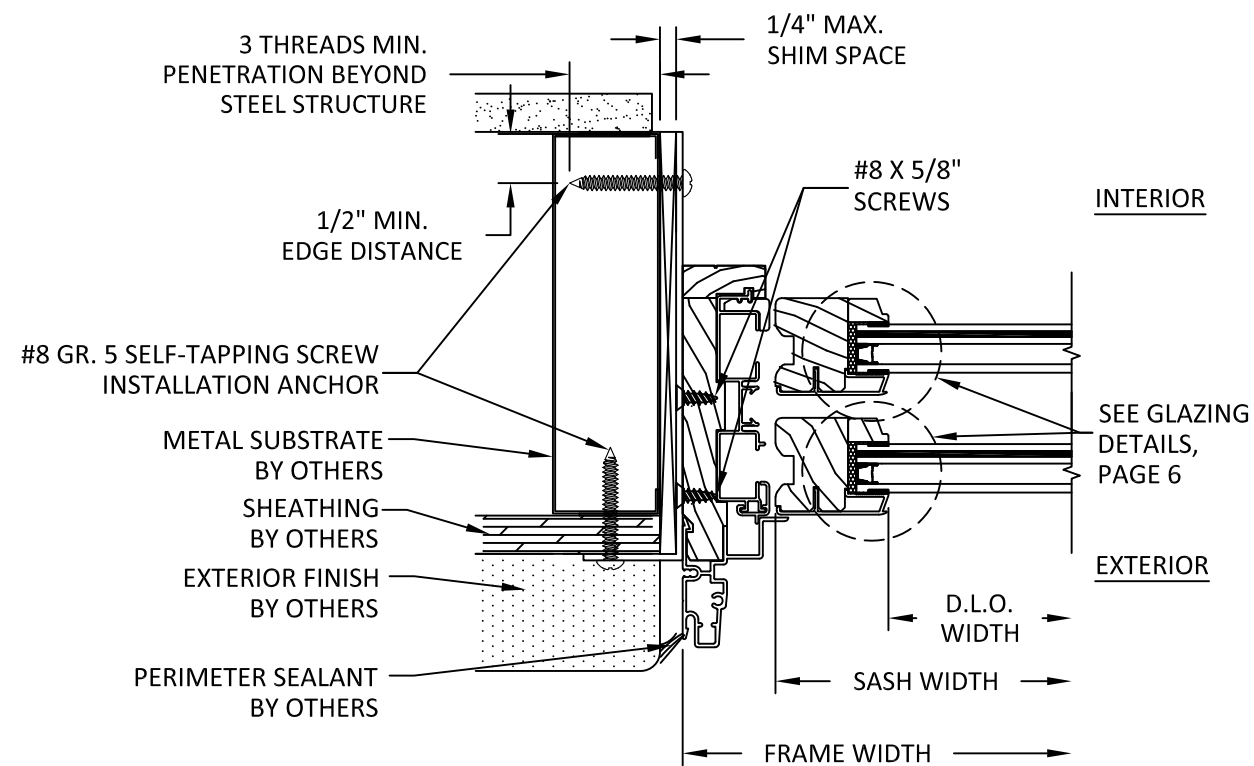
G 4 HORIZONTAL SECTION DH JAMB - STEEL STUD FRAME ALTERNATE CLIP INSTALLATION
